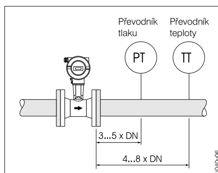
Zabudování měřicího čidla tlaku a teploty
