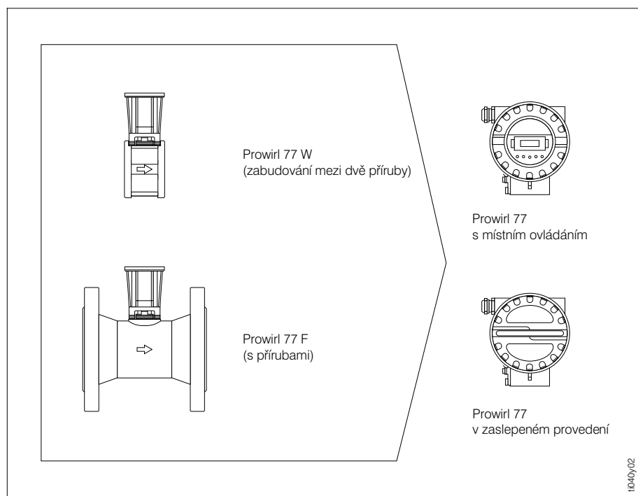
Měřicí systém Prowirl 77
